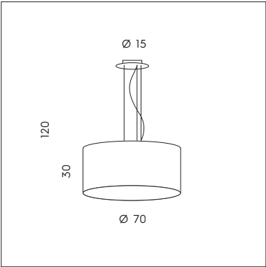
SP 8/503 3 x max 77W E27 CE IP20
