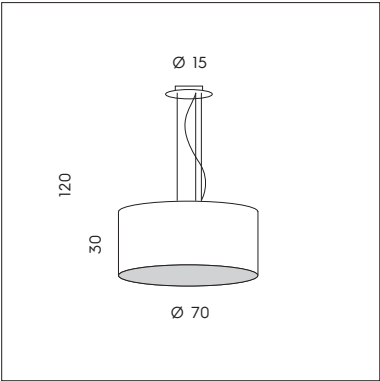
SP 8/503-L 3 x max 77W E27 CE IP20
