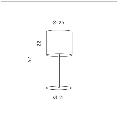
LT 1/503 1 x max 77W E27 CE IP20
