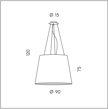
SP 8/505-L 3 x max 77W E27 CE IP20
