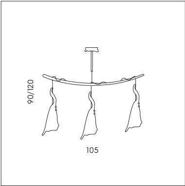
SP S/202 3 x max 46W E14 CE IP20 ▽
