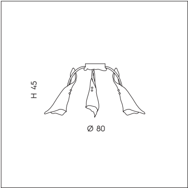
LS Q/202 3 x max 46W E14 CE IP20 ▽
