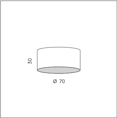
LS 5/503-L 3 x max 77W E27 CE IP20
