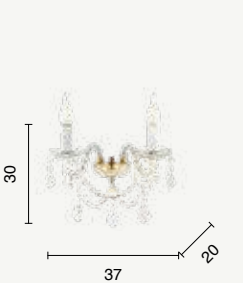
applique wall lamp AP.OPERA/2 AP.OPERA/2-FUMÈ AP.OPERA/2-TORT power: 2 x E14 voltage: 220-230V
