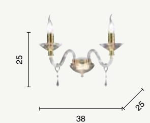
applique wall lamp AP.FIAMMA/2 power: 2 x E14 voltage: 220-230V
